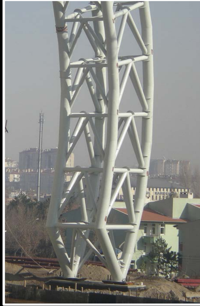
ANA MAKASLARIN KESİTİ : 4.6*8 M , ST52 BORU PROFİL (ÇAP=914 mm , KALINLIK=12-16 mm)
